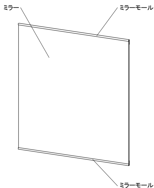
1面鏡 (間口60・61・75・76・90・91cm)
