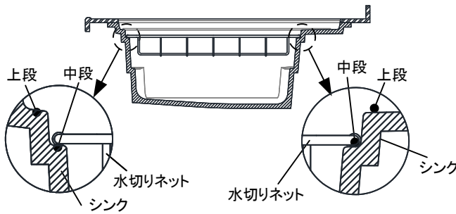
[シンクと水切りネットの断面]
