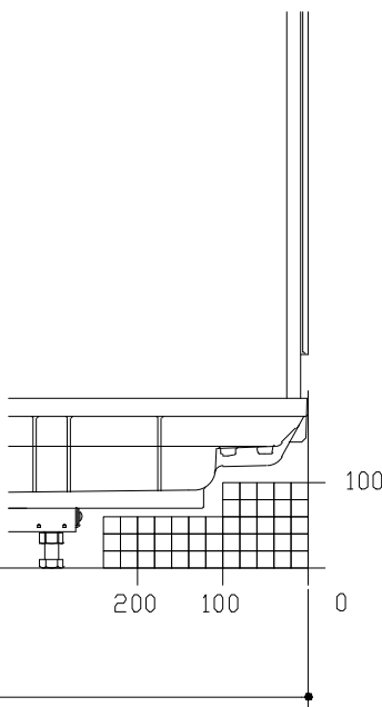
F矢視
