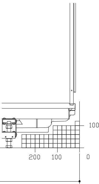
D矢視
