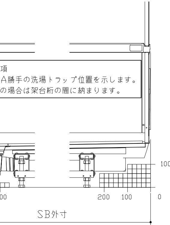
C矢視
