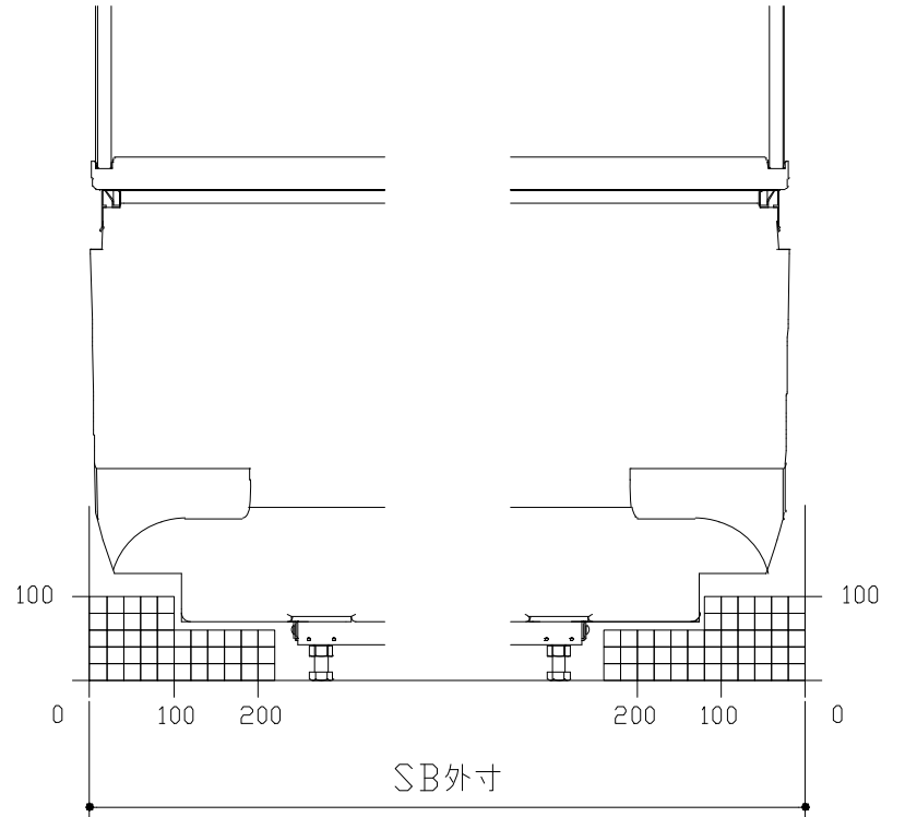
F矢視
