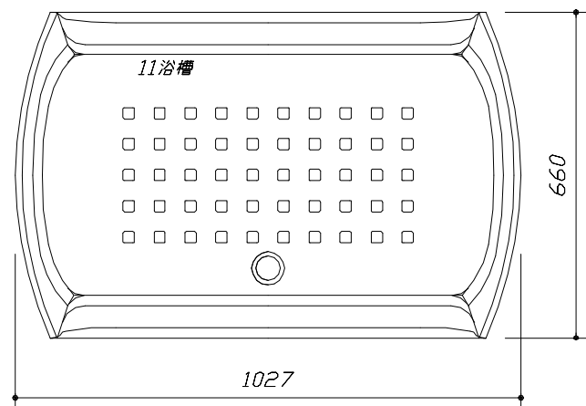
< 浴槽詳細図 >
