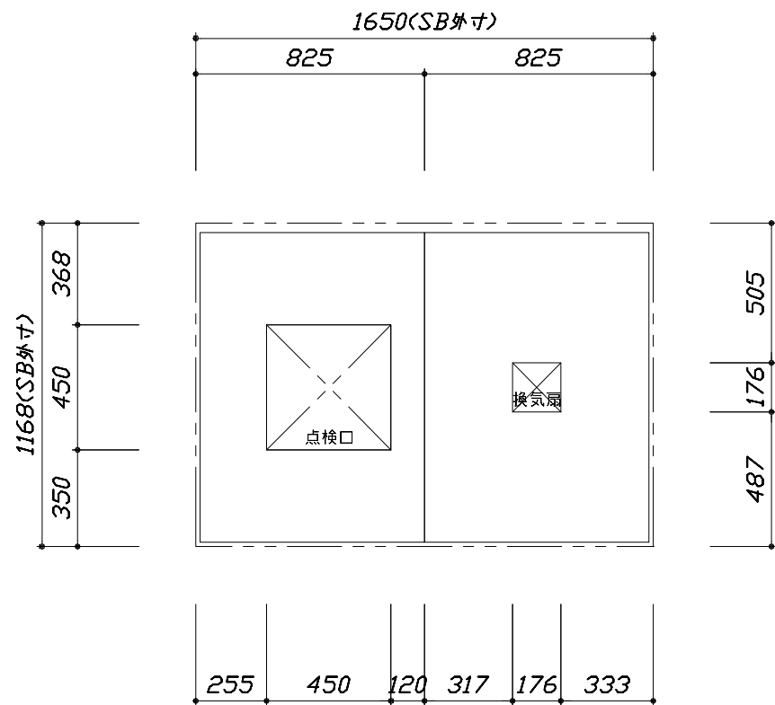
< 天井伏図 >
