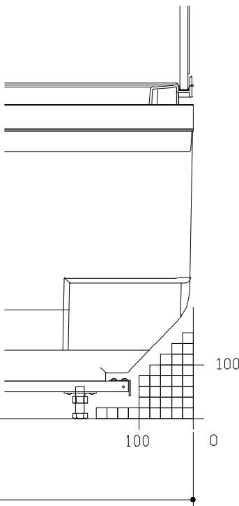
A矢視
