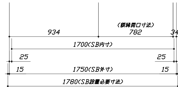
< 平面図 >
