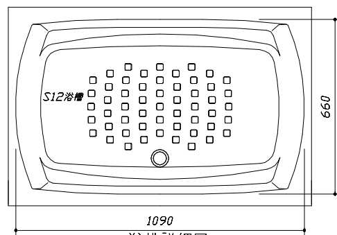
<浴槽詳細図>
