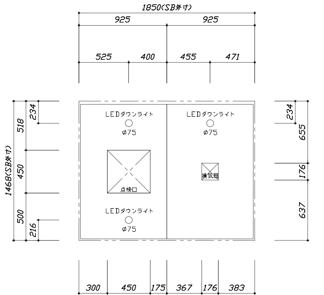
<天井伏図>
