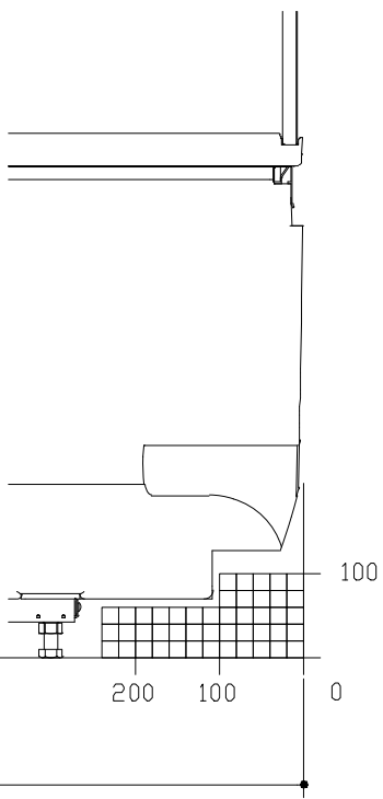
F矢視
