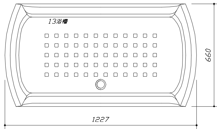
< 浴槽詳細図 >
