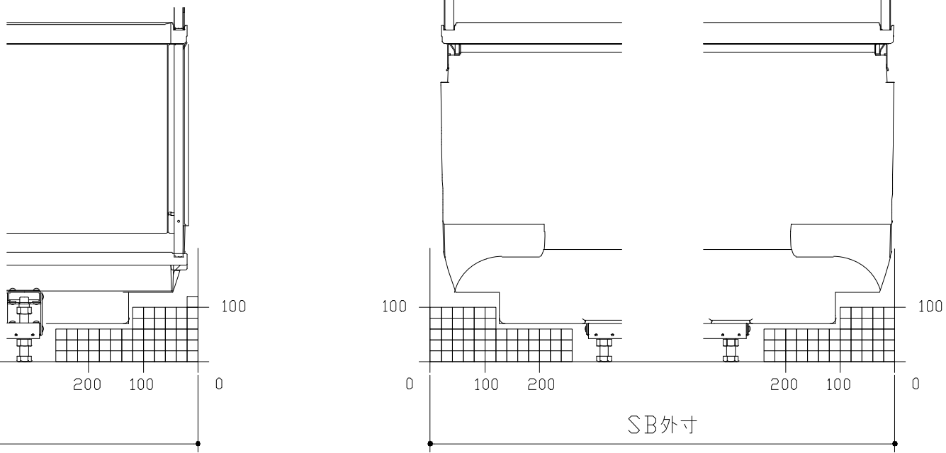
D矢視
