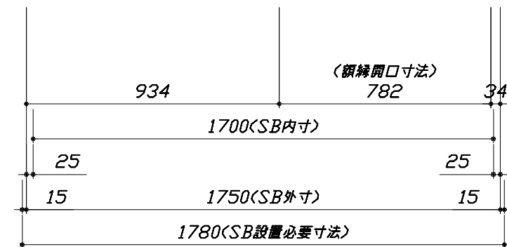
<平面図>
