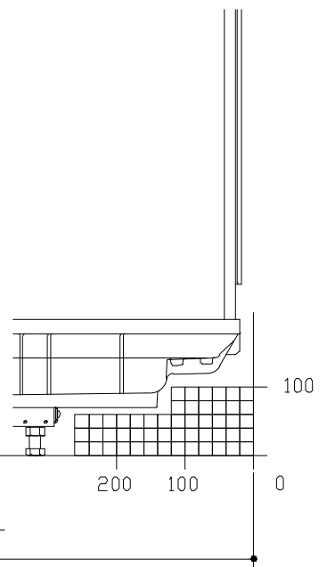
E矢視
