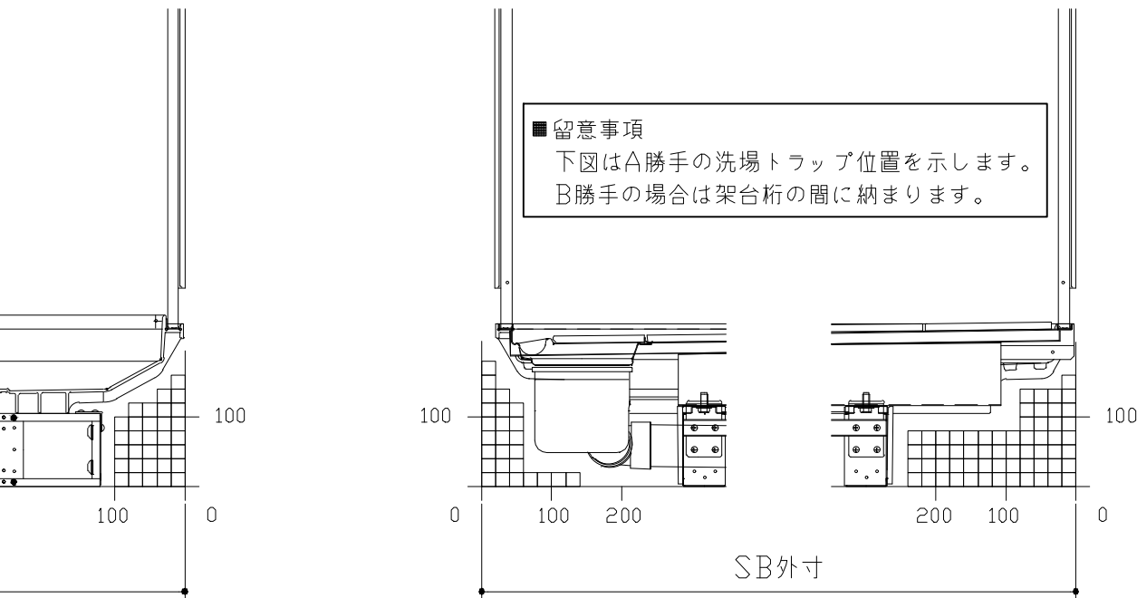
D矢視
