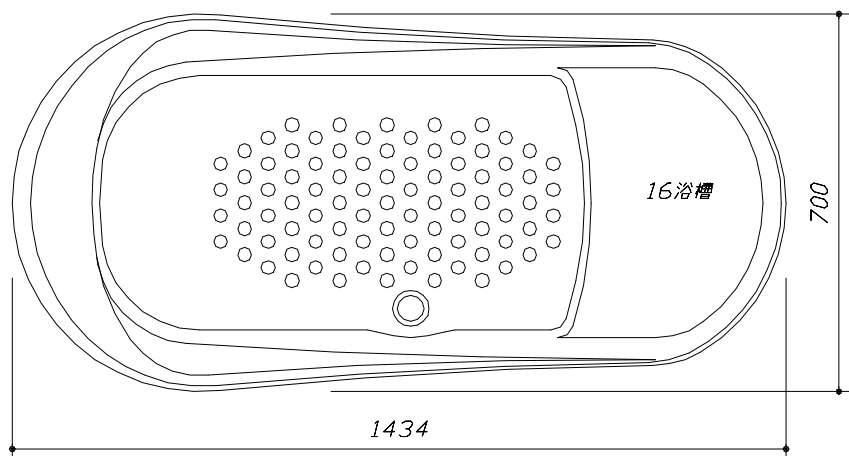
<浴槽詳細図>
