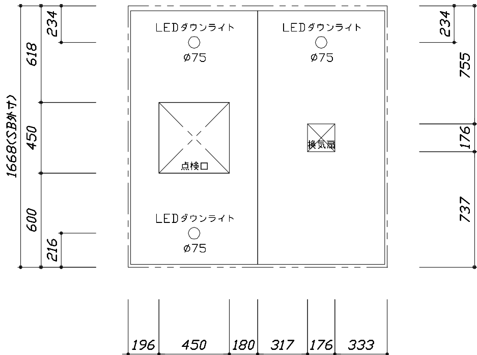
<天井伏図>
