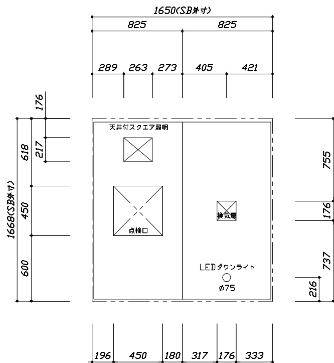
<天井伏図>
