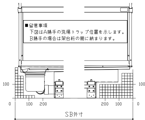
D矢視
