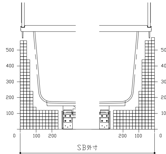
F矢視
