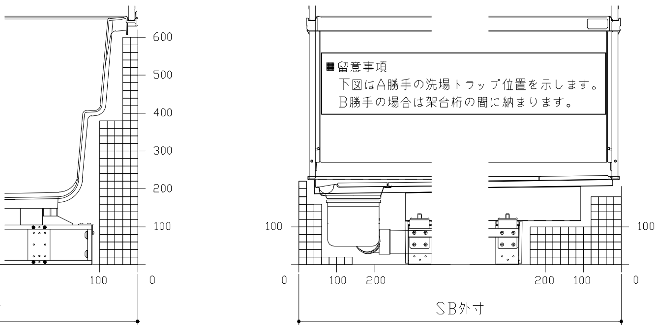
D矢視
