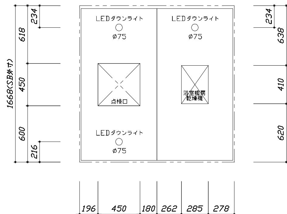
<天井伏図>
