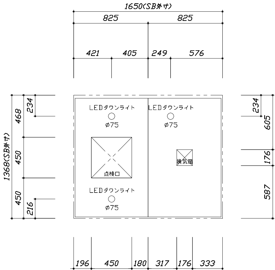
< 天井伏図 >
