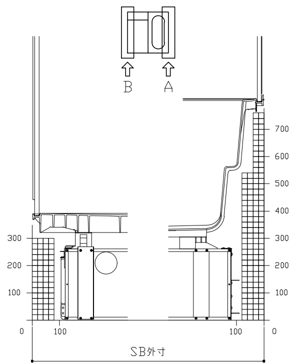
B矢視
