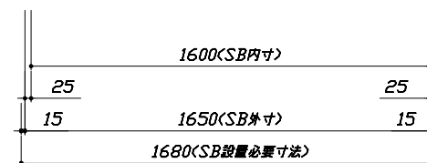
<平面図>
