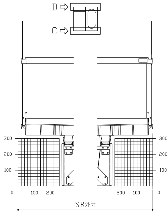
D矢視
