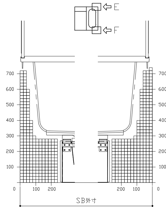
F矢視
