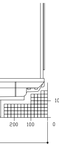
E矢視
