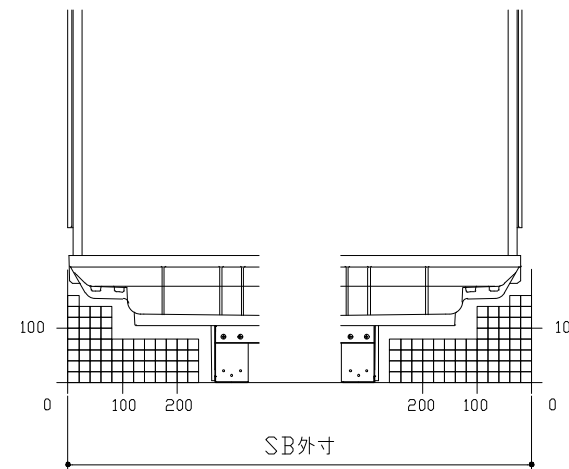
F矢視
