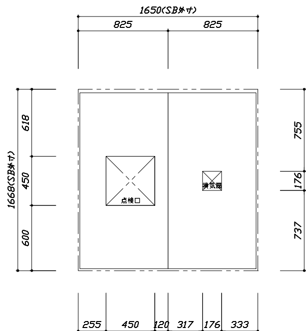
<天井伏図>
