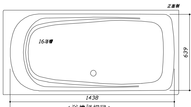
<浴槽詳細図>
