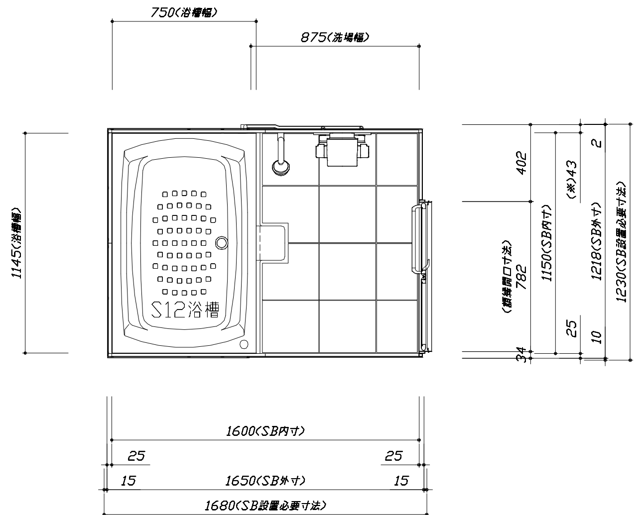
< 平面図 >
