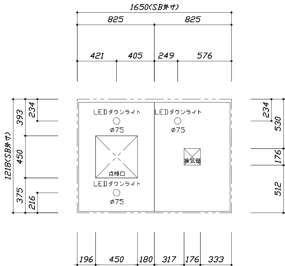
< 天井伏図 >
