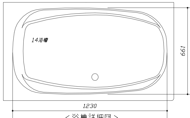
<浴槽詳細図>
