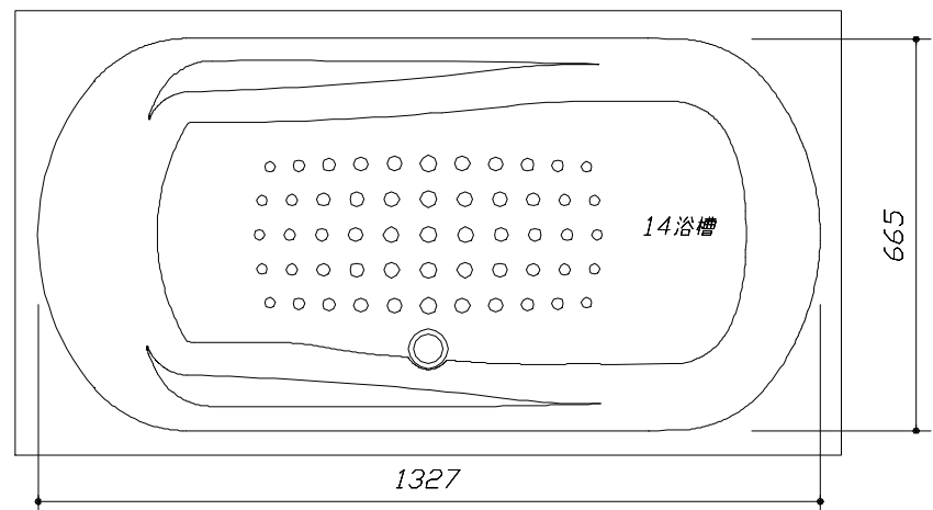
< 浴槽詳細図 >
