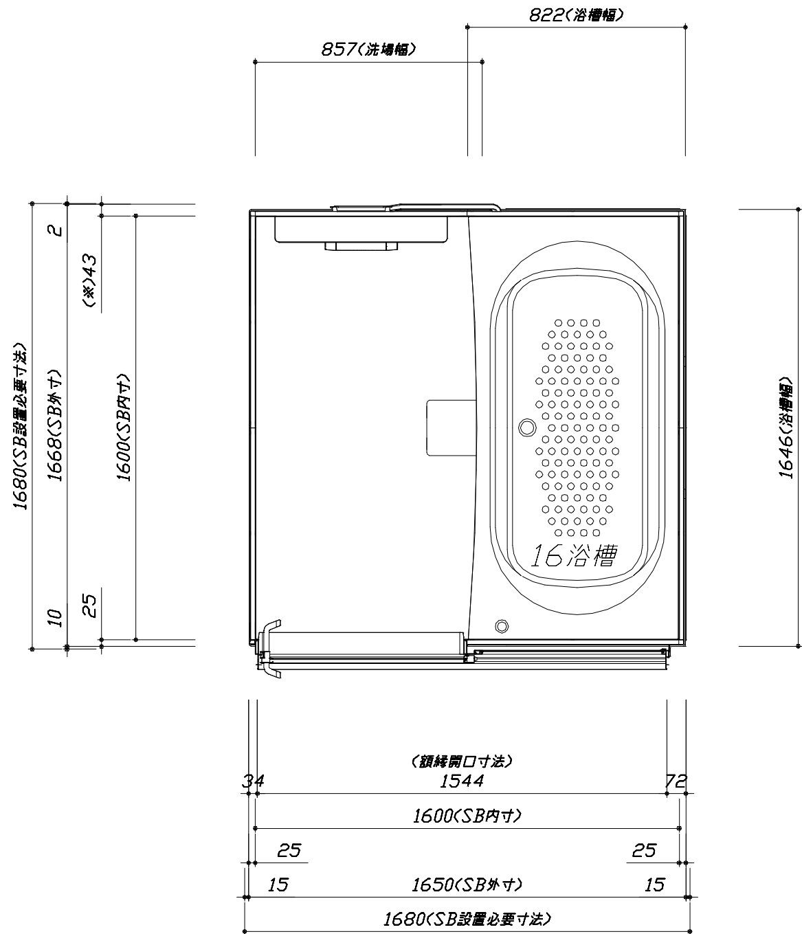
<平面図>
