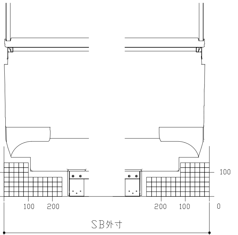
F矢視
