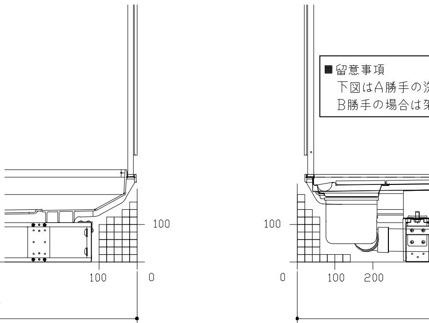
A矢視
