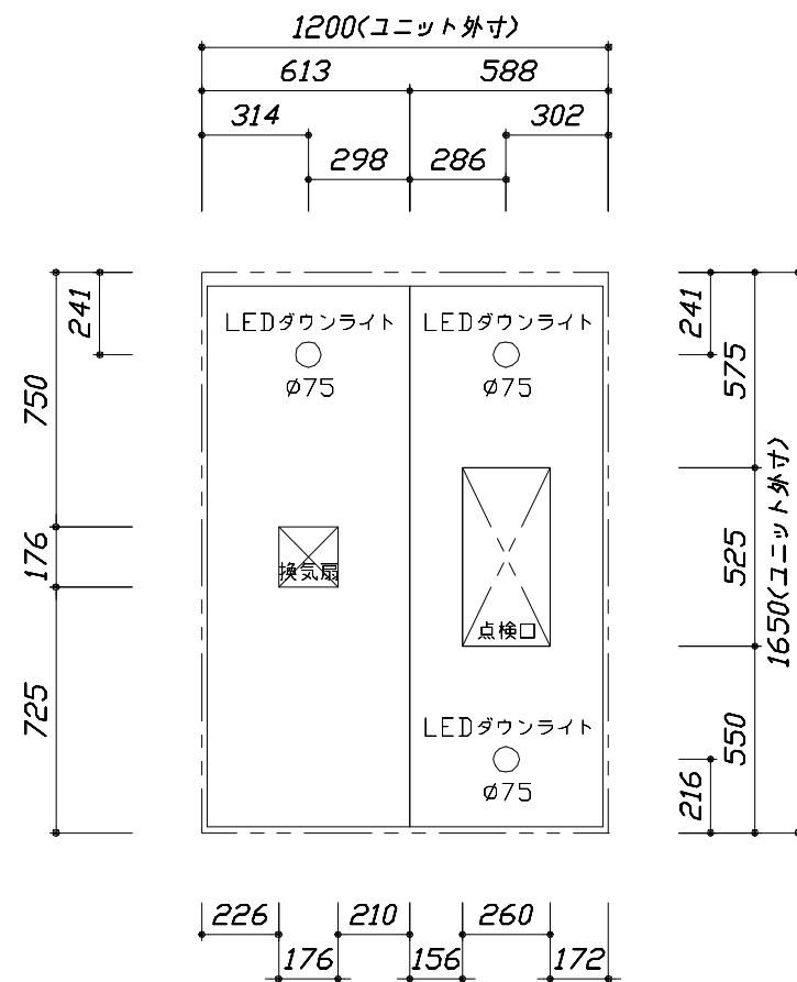
< 天井伏図 >
