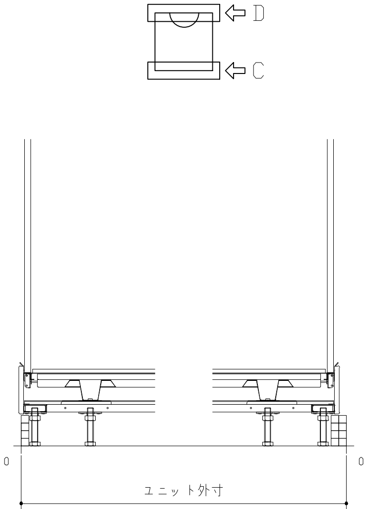
C矢視
