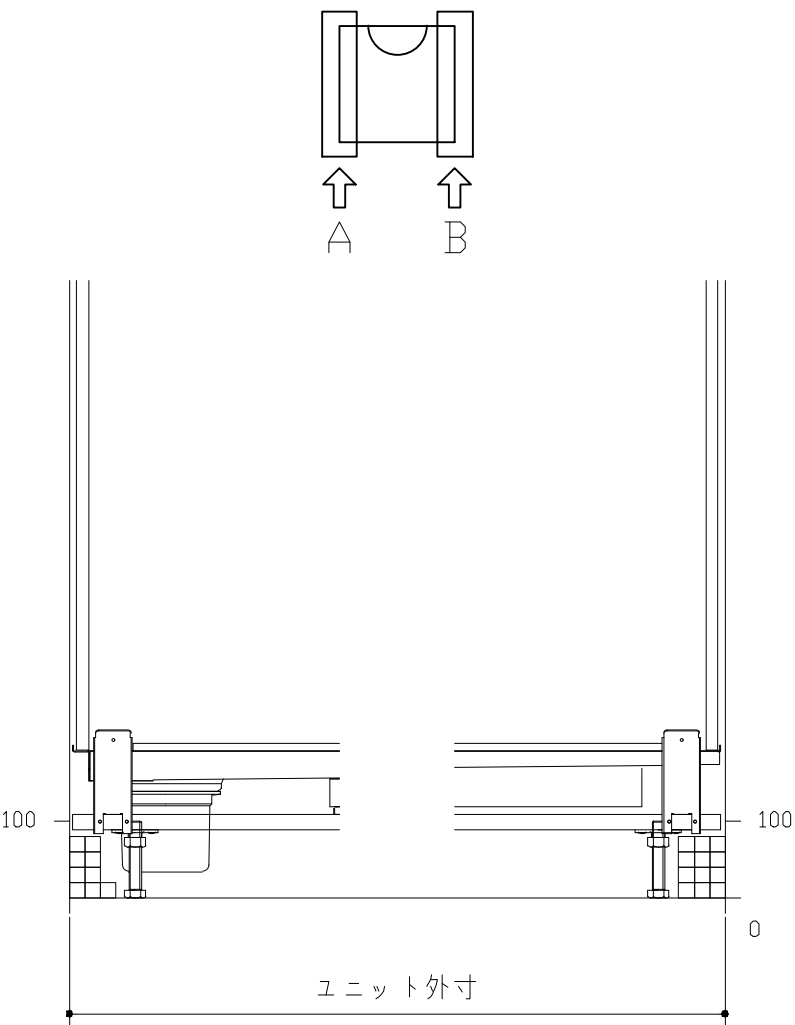
A矢視
