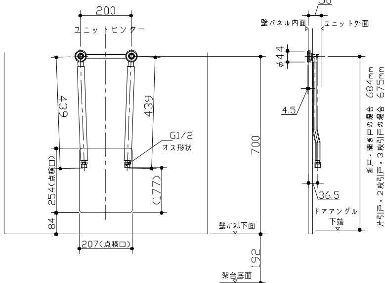
＜給水給湯管取合詳細図＞
