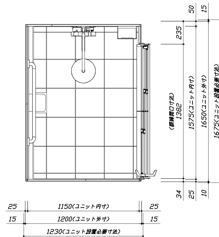
< 平面図 >
