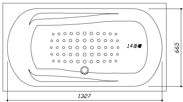
< 浴槽詳細図 >
