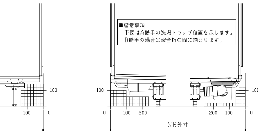
C矢視
