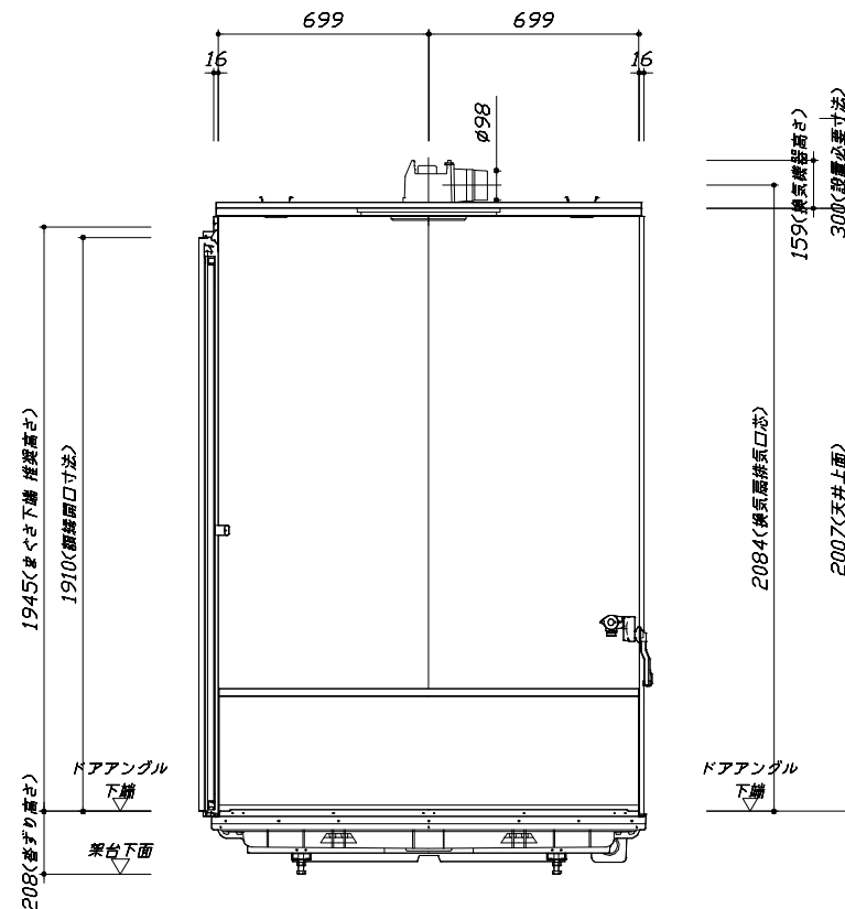
< 浴槽側面図 >
