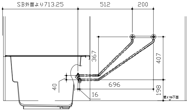
＜給水給湯管取合詳細図＞
