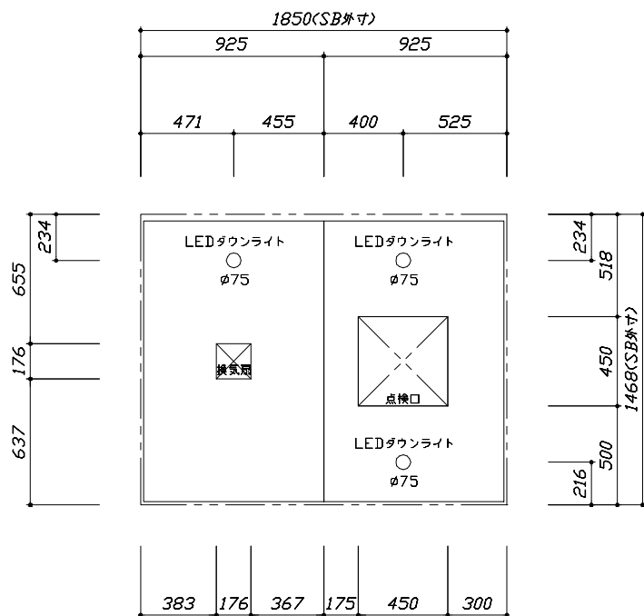
< 天井伏図 >
