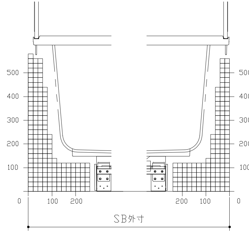
E矢視
