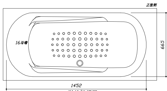
< 浴槽詳細図 >
