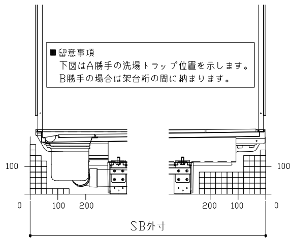
D矢視
