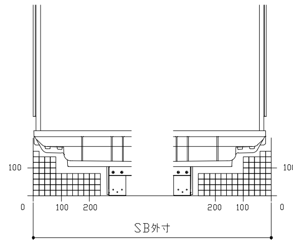
F矢視
