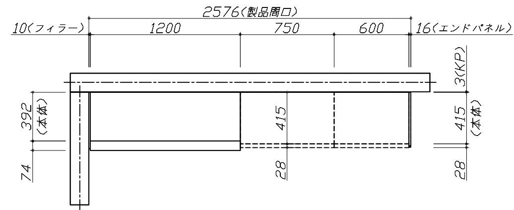
上台伏せ図
