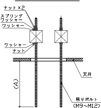
吊ボルト 取付参考図
