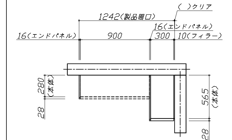
上台伏せ図
