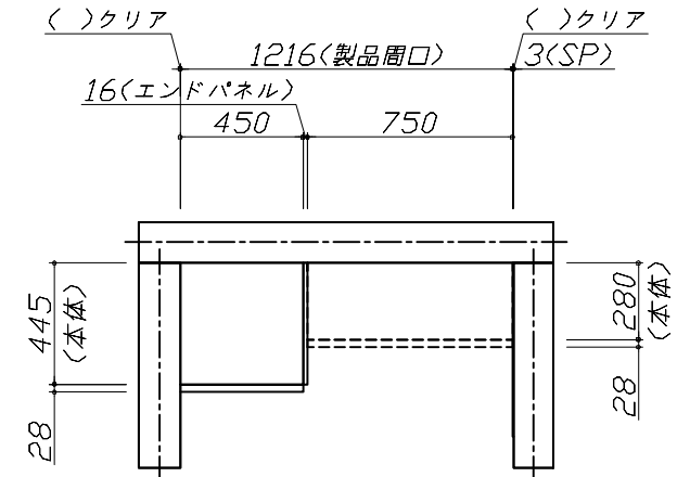
上台伏せ図
